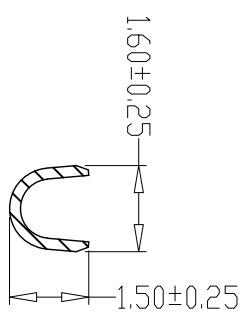
SEC: B-B
